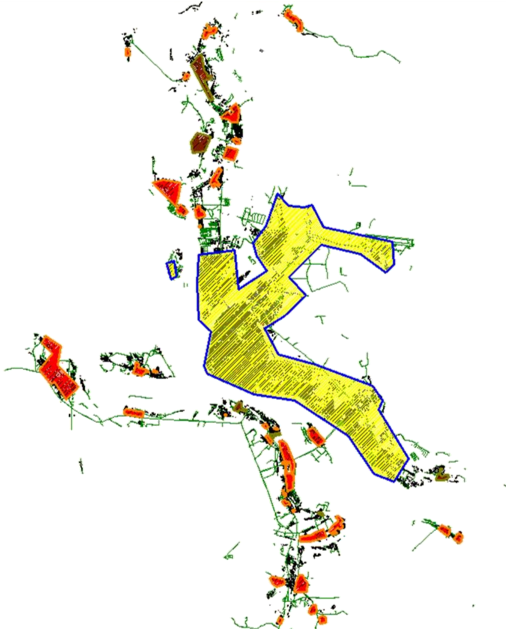
Рисунок 3.1 – Зоны действия энергоисточников г. Архангельска по состоянию базового периода разработки схемы теплоснабжения
