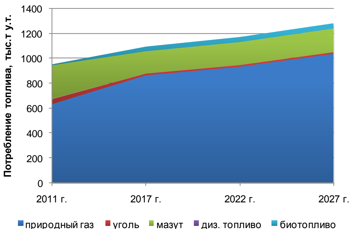
Рисунок 7.1 – Изменение потребления топлива энергоисточниками города по видам топлива
