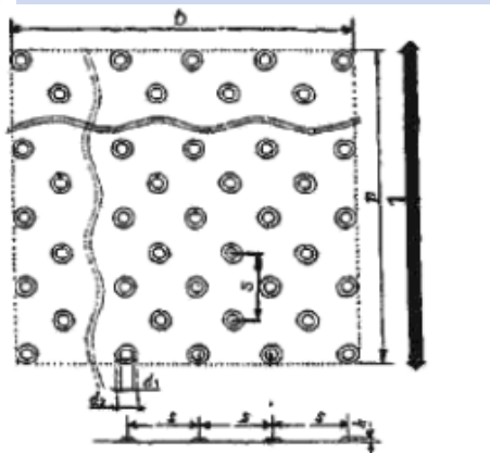
а) Параллельно основному направлению передвижения
