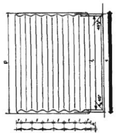
а) Прямые ребра с синусоидальным профилем параллельные основному направлению передвижения
