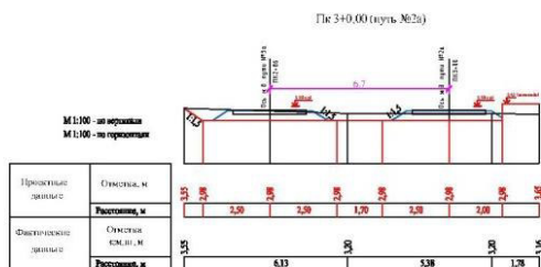
Схема вертикальной планировки Поперечный профиль
